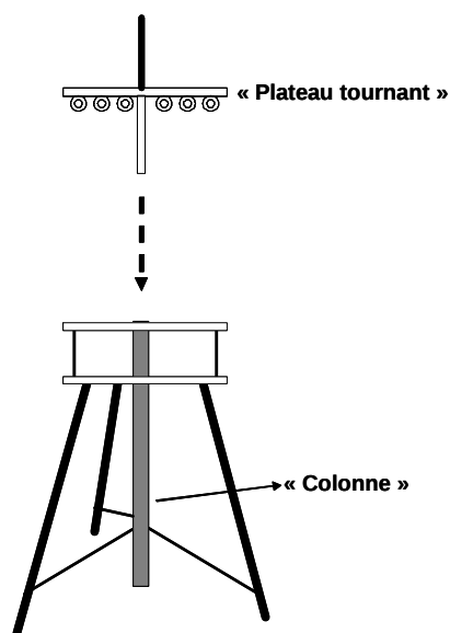
Figure 17 Axe du plateau tournant dans la colonne
