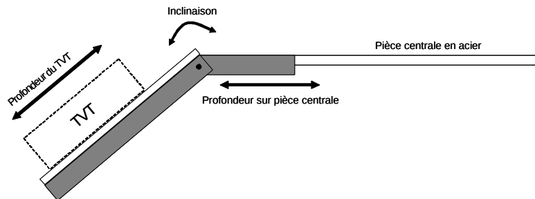
Figure 21 Plan incliné réglable
