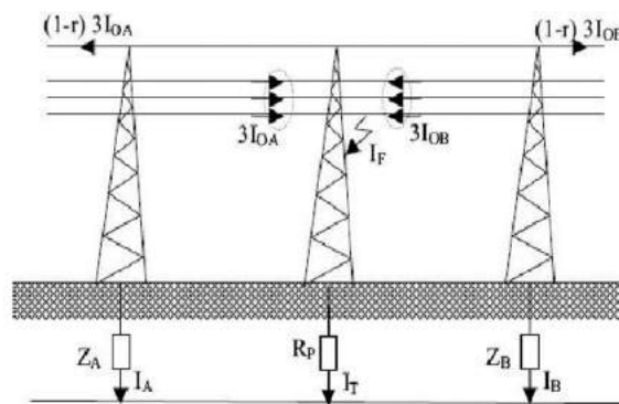
Instalación cable de guarda en torretas
