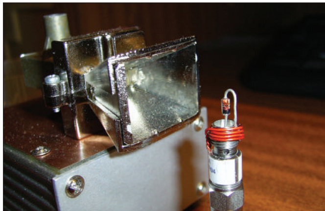
Figura 11: Situación del generador de armónicos delante de la cavidad para proceder a los ajustes de frecuencia.
