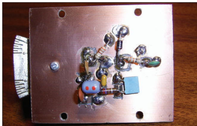
Figura 4: Para la realización de la parte de radiofrecuencia se ha utilizado una placa de circuito impreso virgen a la cual se le han realizado una serie de topes para realizar las conexiones de los diferentes componentes.
