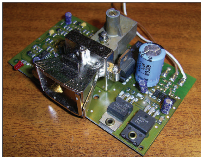
Figura 1: Módulo Doppler en 24 GHz, utilizado en sensores de movimiento.
