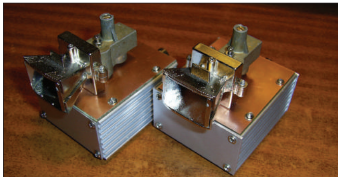
Figura 8: La pareja de transceptores terminados y listos para el QSO.
