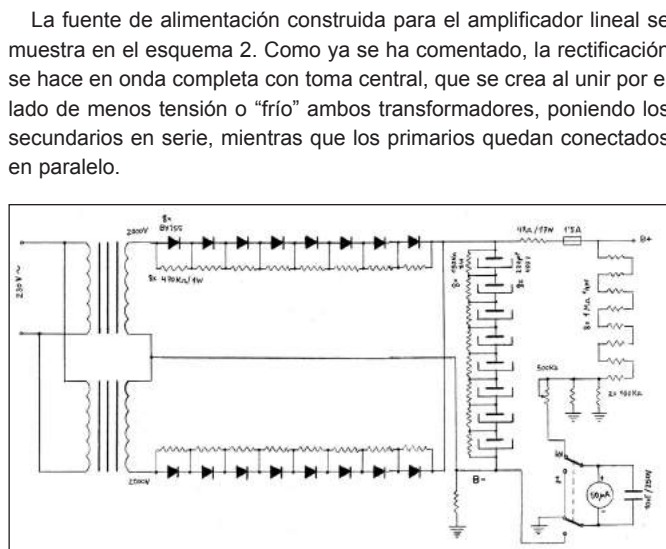
ESQUEMA 2: Fuente de alimentación de alta tensión.
