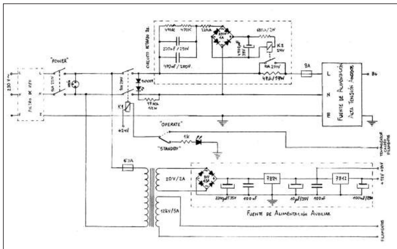
ESQUEMA 4: Circuito de alimentación de red.
