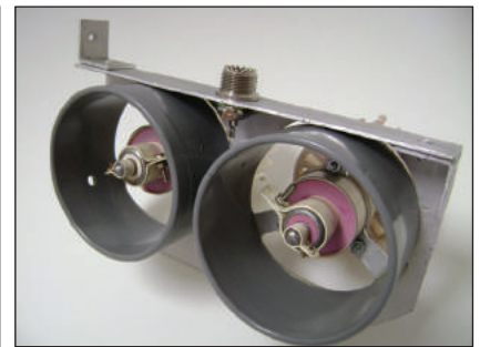
FOTO 9: Soporte de los triodos vista trasera.
